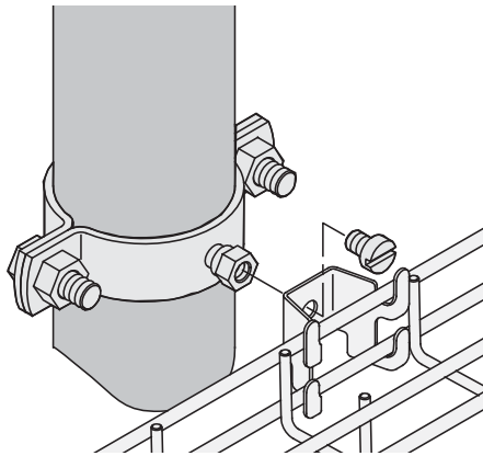
S162 Rohraufhängung
