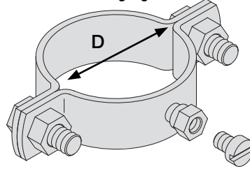
S162 Rohraufhängung
