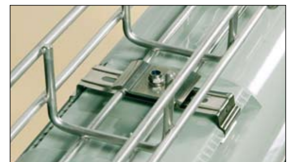
S41M Klemmplatte
